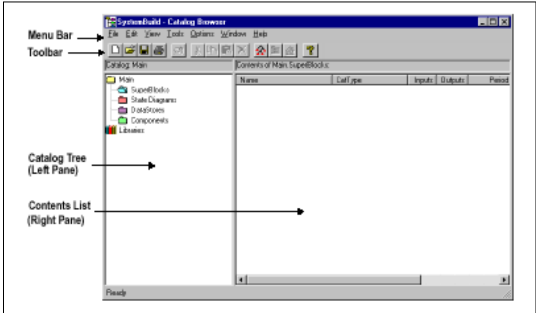
Figure 4-1. Catalog Browser
